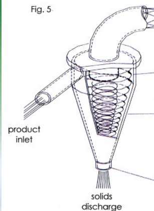
2HY-PZ Hydrozyklon mit Feststoffaustrag
