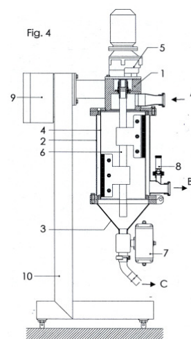
SFR Vorfilter mit Feststoffaustrag
